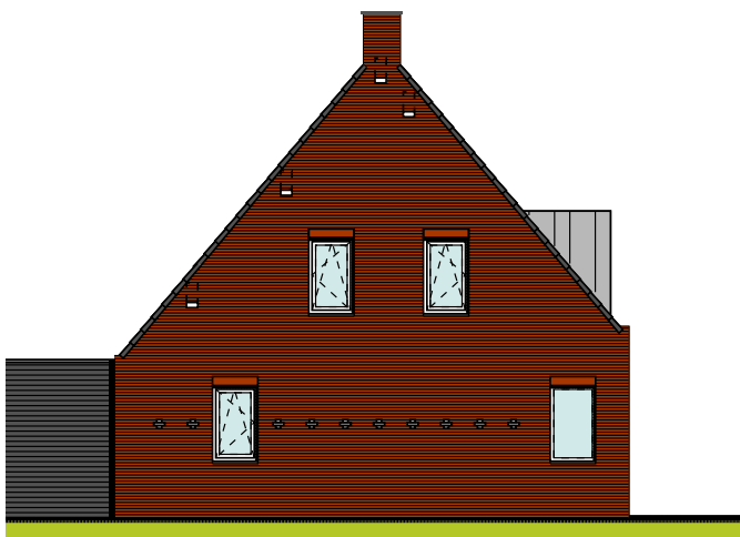
Linkergevel
